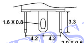
16mm B Solder Lug
